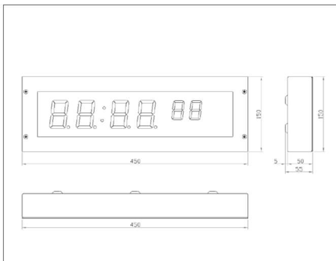
einseitige Ausführung
