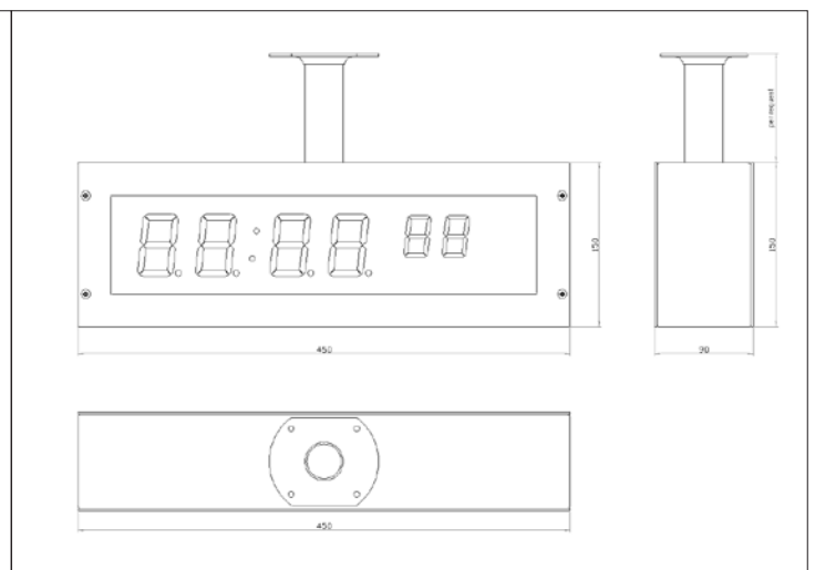
doppelseitige Ausführung
